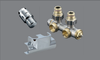
R+F Optiline-Anschluss-Set für Badheizkörper
